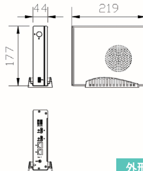
外形図
