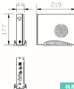
外形図
