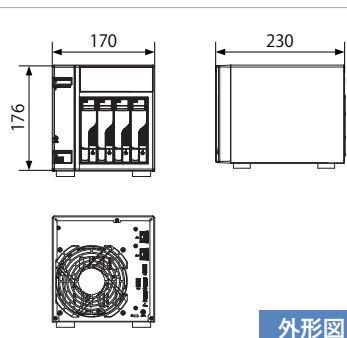
外形図
